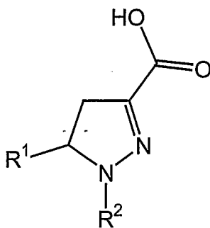
(VI)
