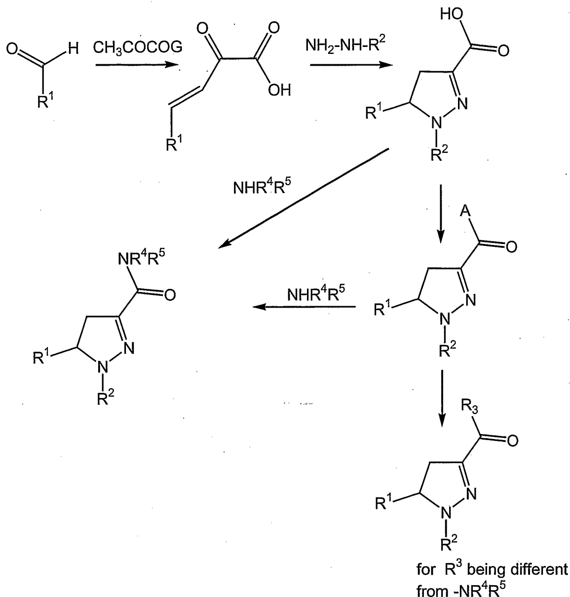
Scheme I:
