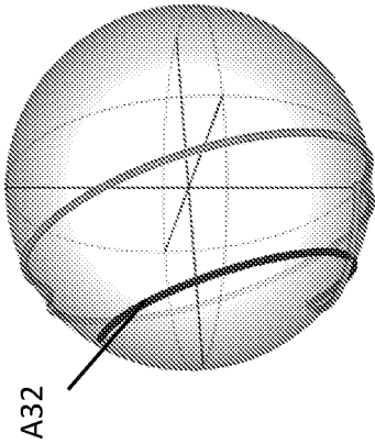
Bloch sphere A32
