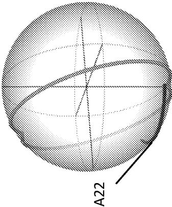
Bloch sphere A22
