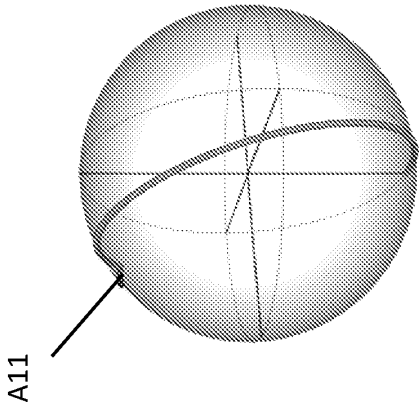
Bloch sphere A11
