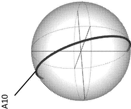
Bloch sphere A10
