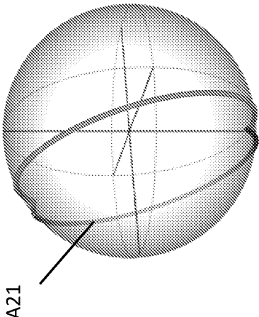
Bloch sphere A21
