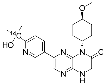
14 C-Compound A.
