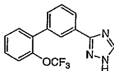
3-[3-(2-Trifluoromethoxyphenyl)-phenyl]-1,2,4-triazole
