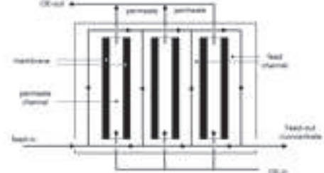
1. plate-and-frame module (3 modules)
