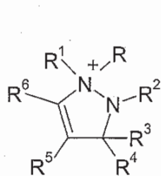
(IVk)
