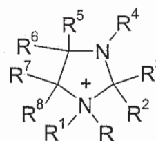
(IVt)
