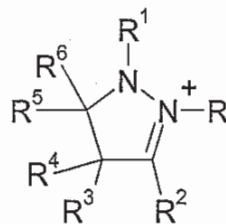
(IVj)
