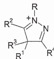
(IVh)
