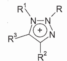
(IVr')
