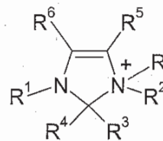
(IVl)
