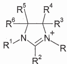
(IVm)
