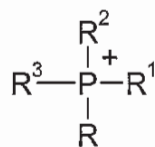
(IVx)
