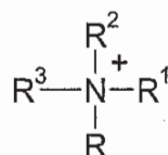
(IVu)
