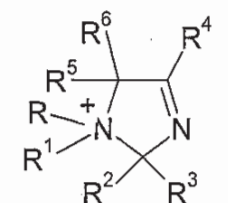
(IVn')
