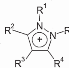
(IVf)
