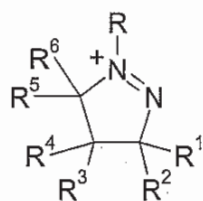
(IVi)
