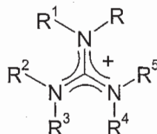
(IVv)
