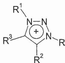
(IVr'')
