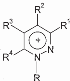
(IVb)
