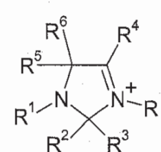
(IVn)
