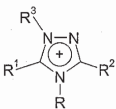
(IVq'')
