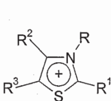
(IVo)
