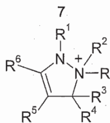
(IVk')
