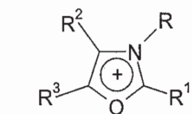
(IVp)
