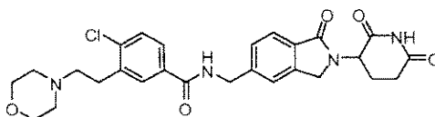
4-chloro-N-((2-(2,6-dioxopiperidin-3-yl)-1-oxoisindolin-5-yl)methyl)-3-(2-morpholinoethyl)benzamide;
