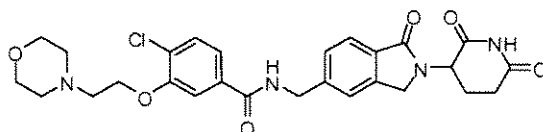
4-chloro-N-((2-(2,6-dioxopiperidin-3-yl)-1-oxoisindolin-5-yl)methyl)-3-(2-morpholinoethoxy)benzamide.
