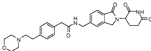
N-((2-(2,6-dioxopiperidin-3-yl)-1-oxoisindolin-5-yl)methyl)-2-(4-(2-morpholinoethyl)phenyl)acetamide;
