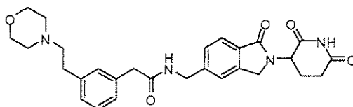
N-((2-(2,6-dioxopiperidin-3-yl)-1-oxoisindolin-5-yl)methyl)-2-(3-(2-morpholinoethyl)phenyl)acetamide;
