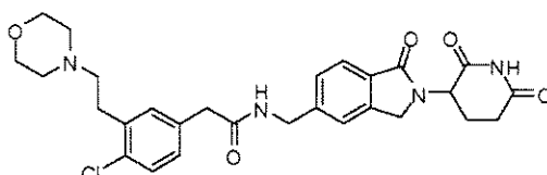
2-(4-chloro-3-(2-morpholinoethyl)phenyl)-N-((2-(2,6-dioxopiperidin-3-yl)-1-oxoisindolin-5-yl)methyl)acetamide;
