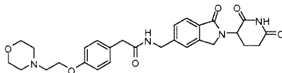
N-((2-(2,6-dioxopiperidin-3-yl)-1-oxoisindolin-5-yl)methyl)-2-(4-(2-morpholinoethoxy)phenyl)acetamide;
