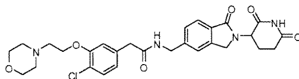
2-(4-chloro-3-(2-morpholinoethoxy)phenyl)-N-((2-(2,6-dioxopiperidin-3-yl)-1-oxoisindolin-5-yl)methyl)acetamide;
