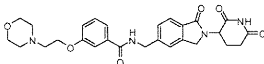
N-((2-(2,6-dioxopiperidin-3-yl)-1-oxoisindolin-5-yl)methyl)-3-(2-morpholinoethoxy)benzamide;
