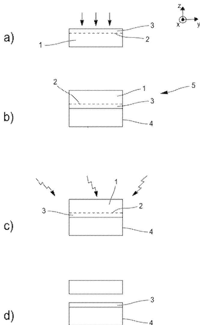
FIG. 1: Art Antérieur
