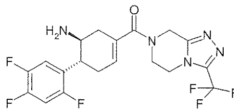
ABT-341
