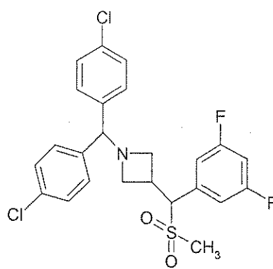
AVE1625
