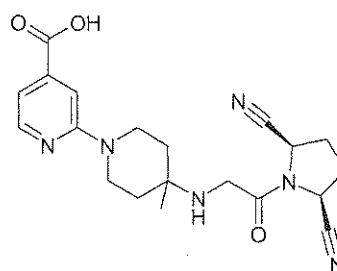
ABT-279
