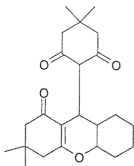
L-152804
