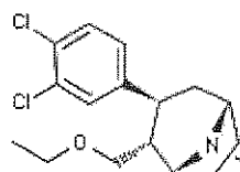
Tesofensine
