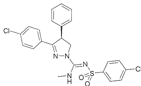
SLV-319
