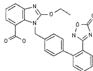
TAK-536
