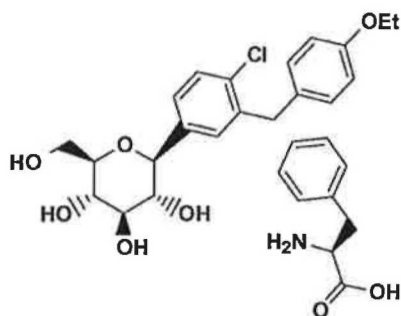
Compound Ik
