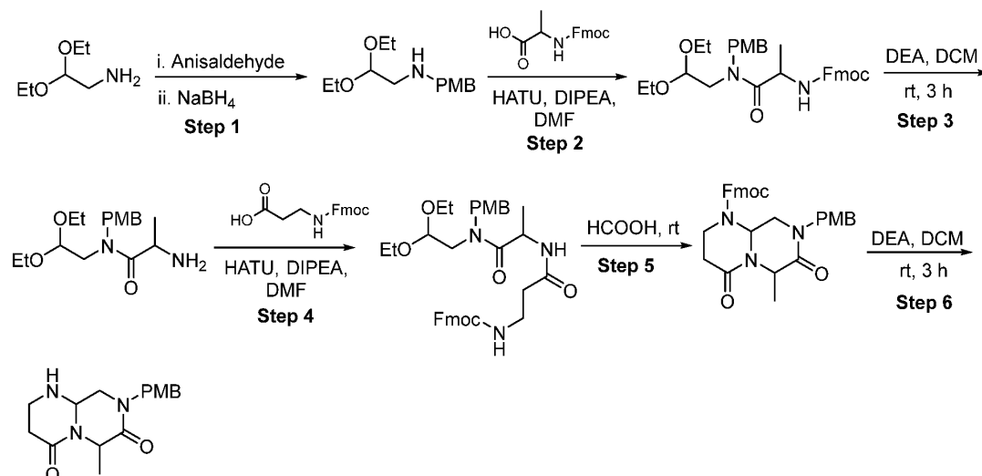
Scheme 14.
