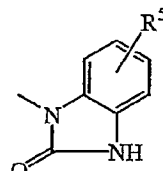
(b-11)
