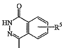
(b-5)
