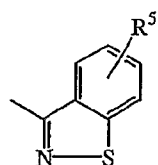
(b-9)
