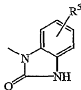
(b-11)
