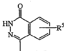
(b-5)
