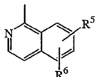
(b-6)
