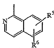
(b-6)
