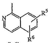
(b-6)
