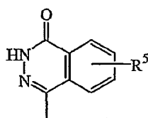
(b-5)
