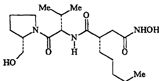
Epiactinonin
