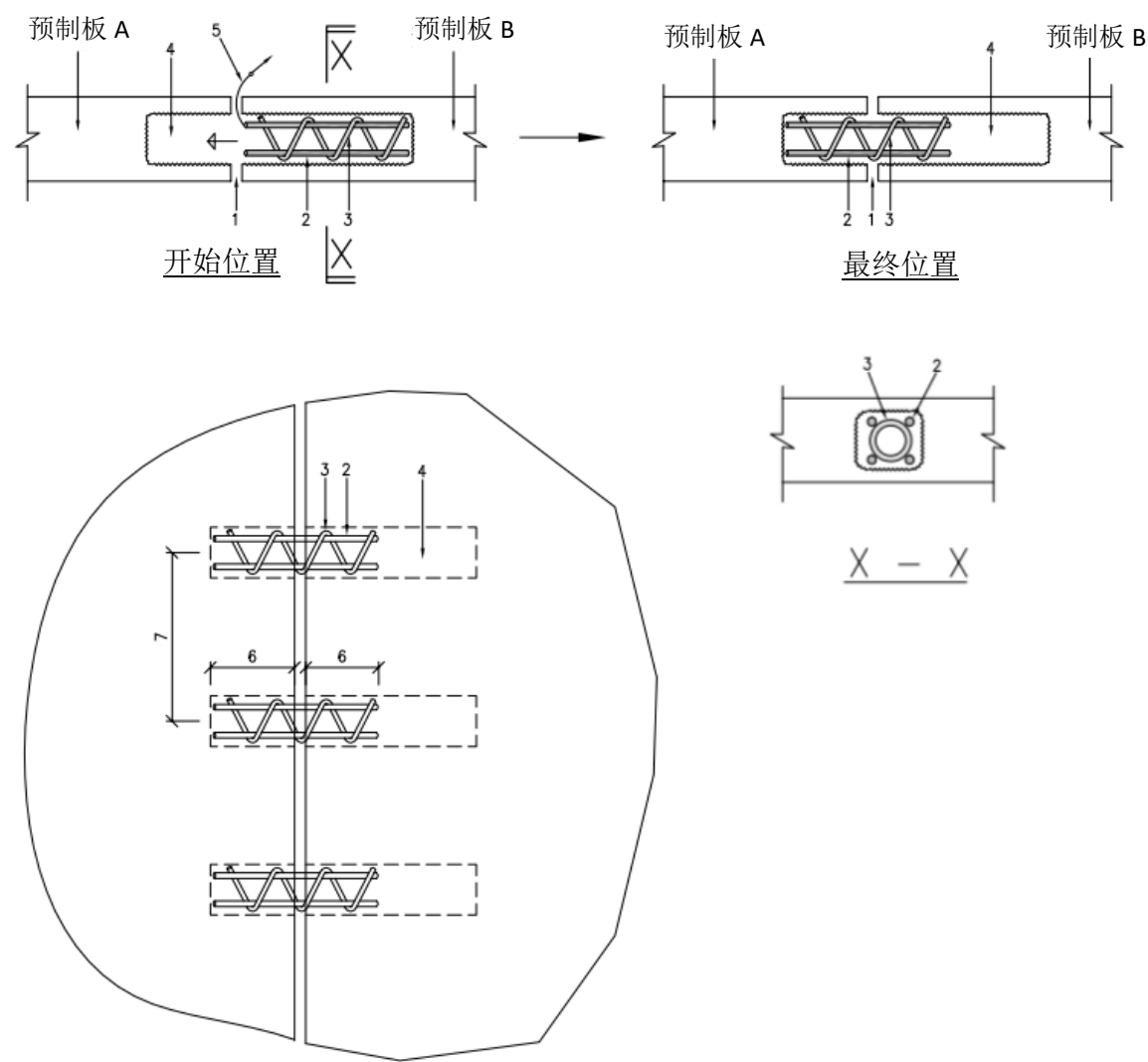
一组以连接螺旋钢筋连接上的预制板的平面图
