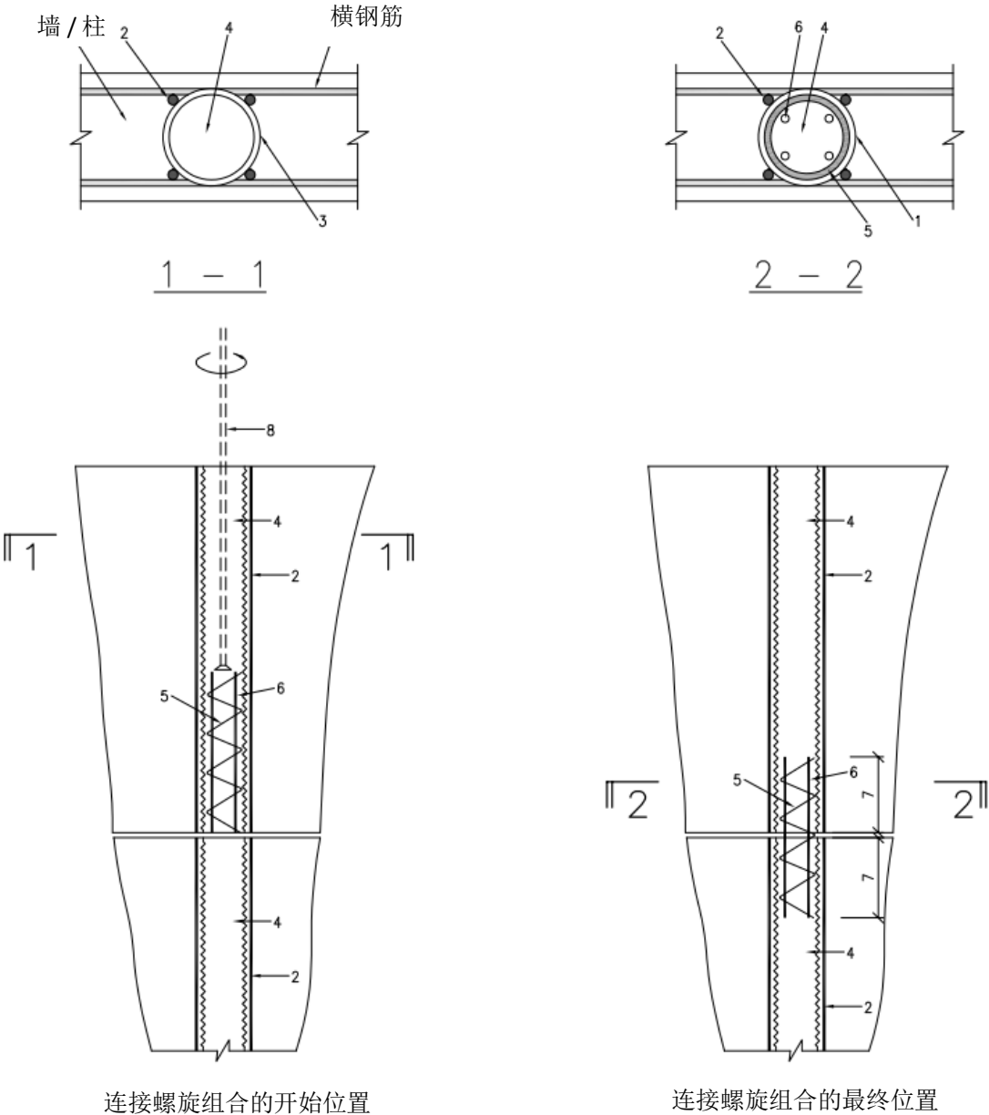
一种以螺旋钢筋组合连接加固墙和柱的方案
