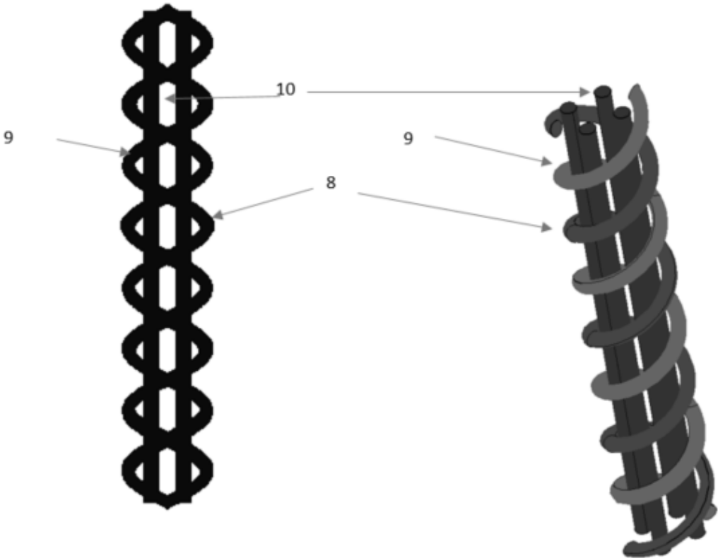
双螺旋钢筋连接件
