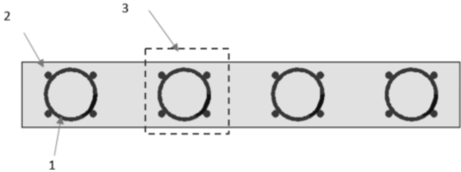
用螺旋钢筋加强的结构墙的俯视图
