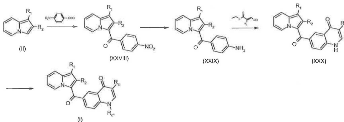
Scheme 7 (Method 7):
