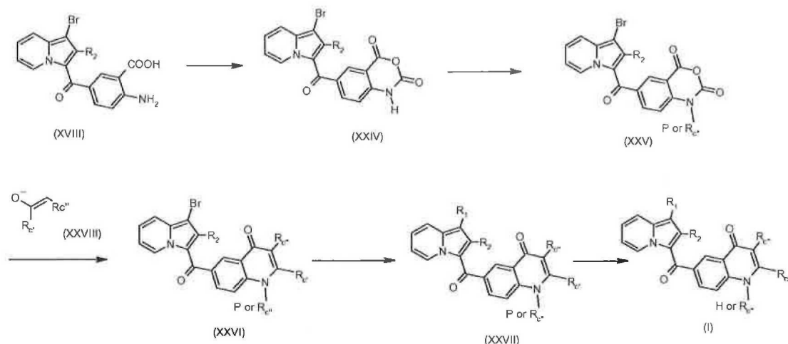
Scheme 6 (Method 6):
