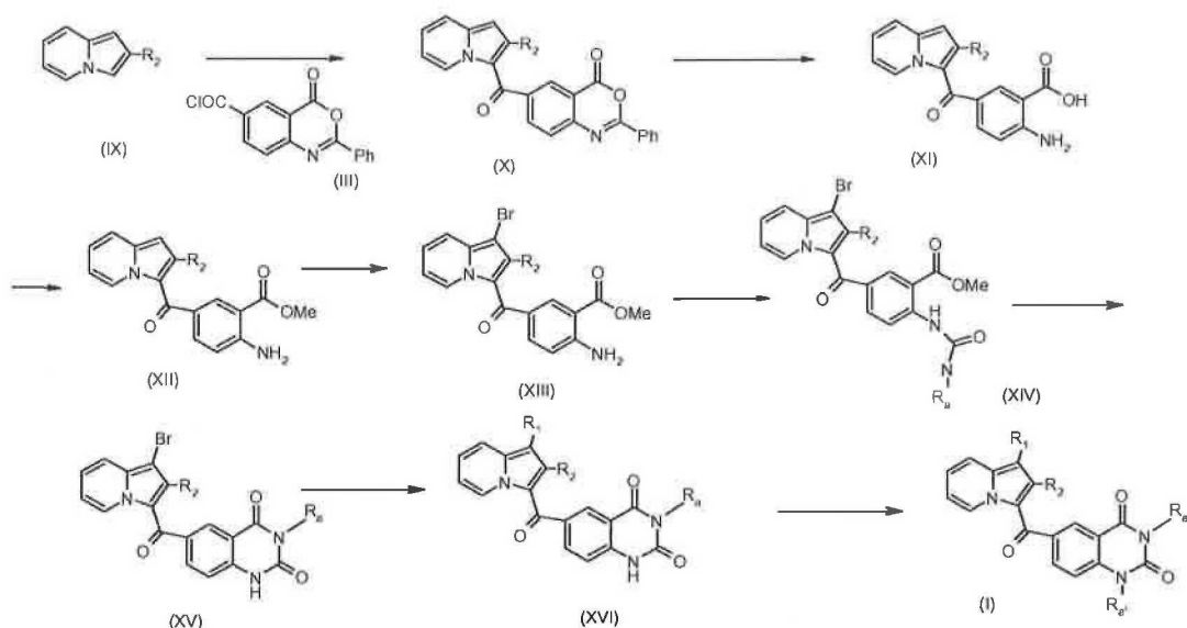
Scheme 2 (Method 2):
