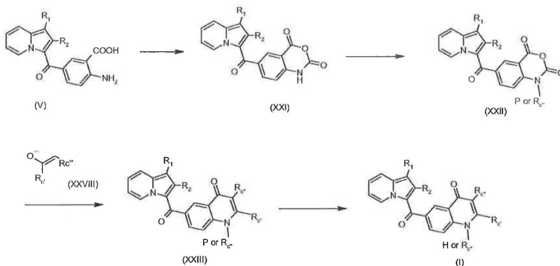
Scheme 5 (Method 5):
