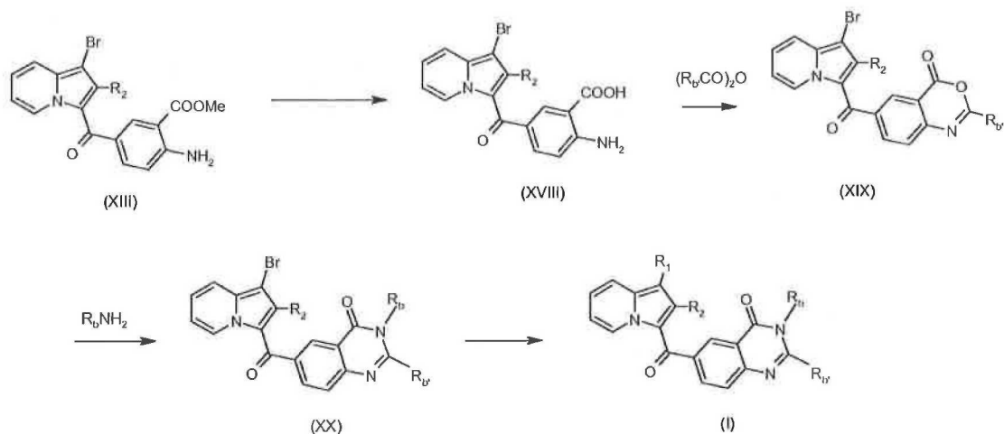
Scheme 4 (Method 4):
