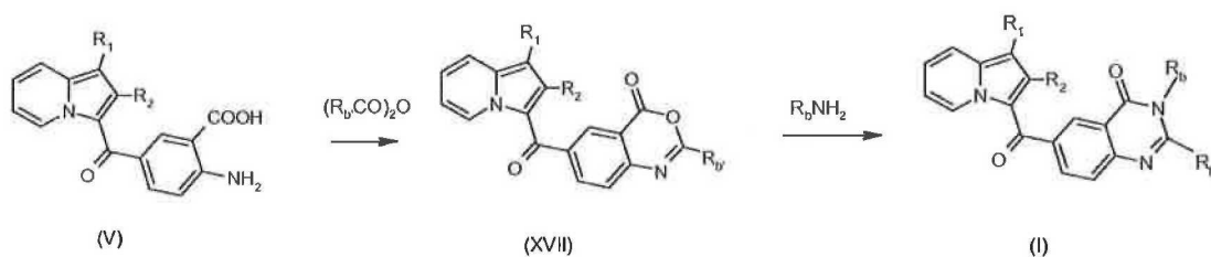
Scheme 3 (Method 3):
