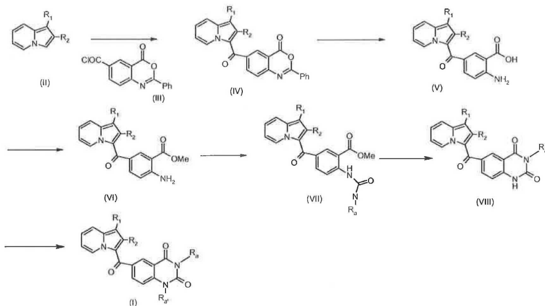
Scheme 1 (Method 1):
