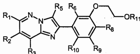
Formula (VI);
