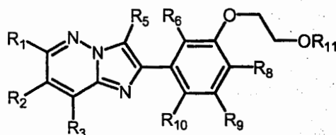
Formula (VI);
