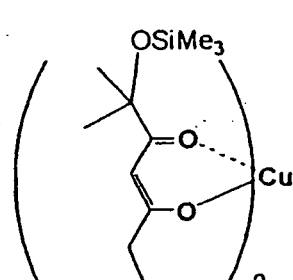
(XI)
