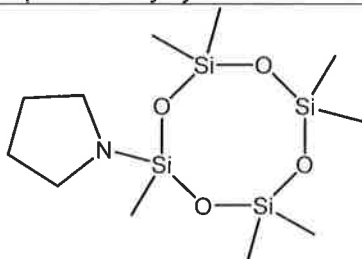
2-pyrrolidino-2,4,4,6,6,8,8-heptamethylcyclotetrasiloxane
