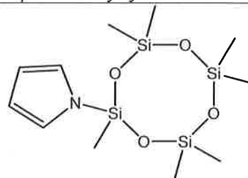
2-pyrrolyl-2,4,4,6,6,8,8-heptamethylcyclotetrasiloxane
