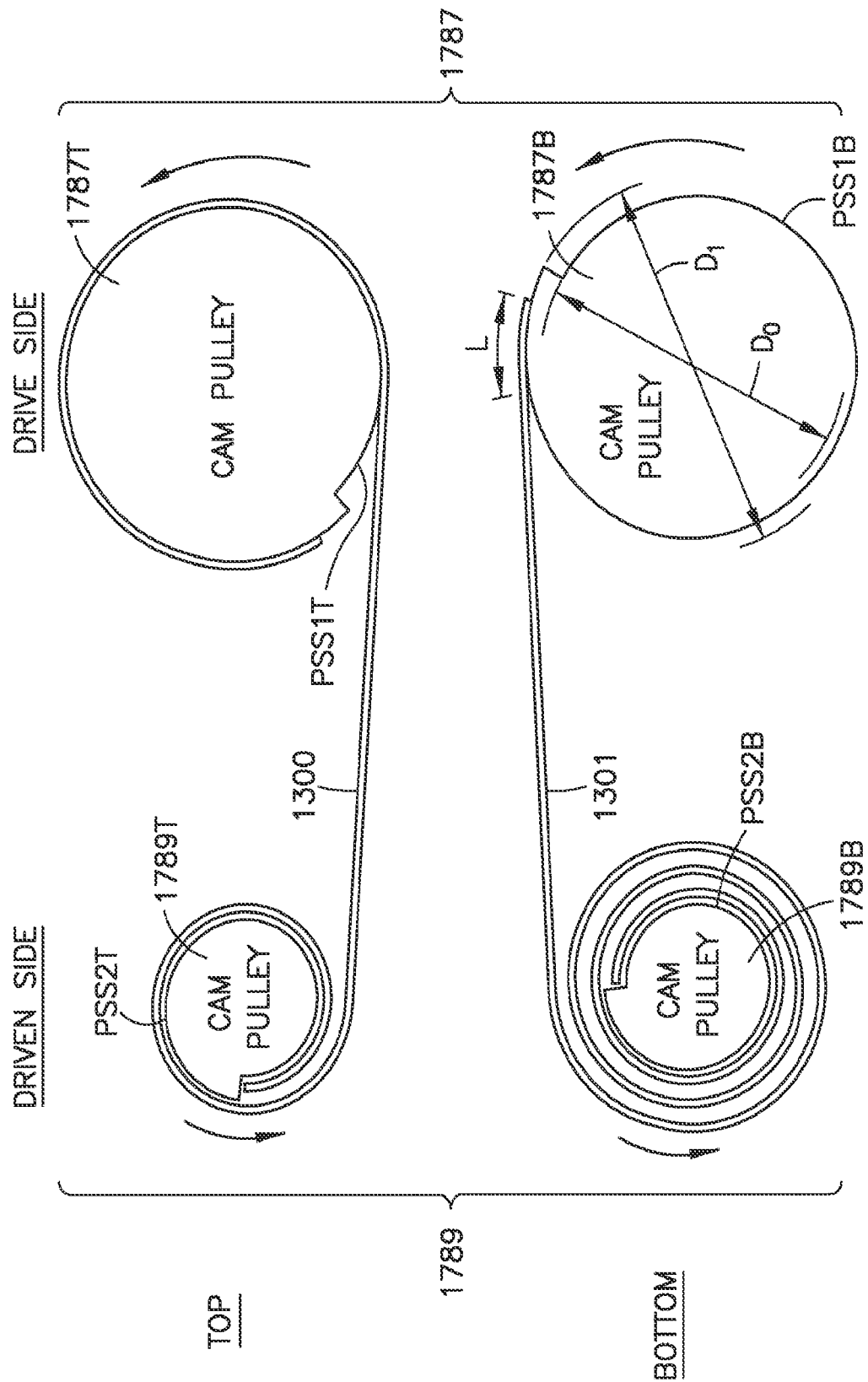
FIG. 13A
