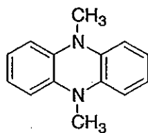
(Me) 2 P
