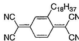
C 18 TCNQ
