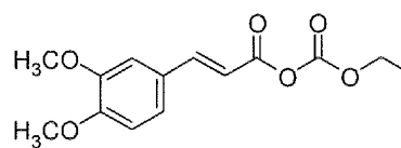
Monomer-3
