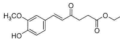
Monomer-6
