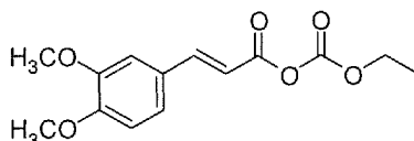
Monomer-3
