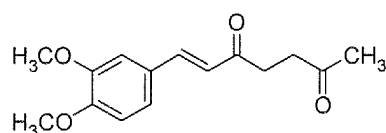
Monomer-7
