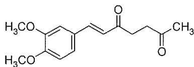
Monomer-7
