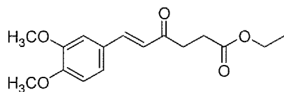
Monomer-5
