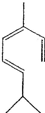
Alloocimene(2)
