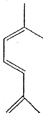
Alloocimene(3)
