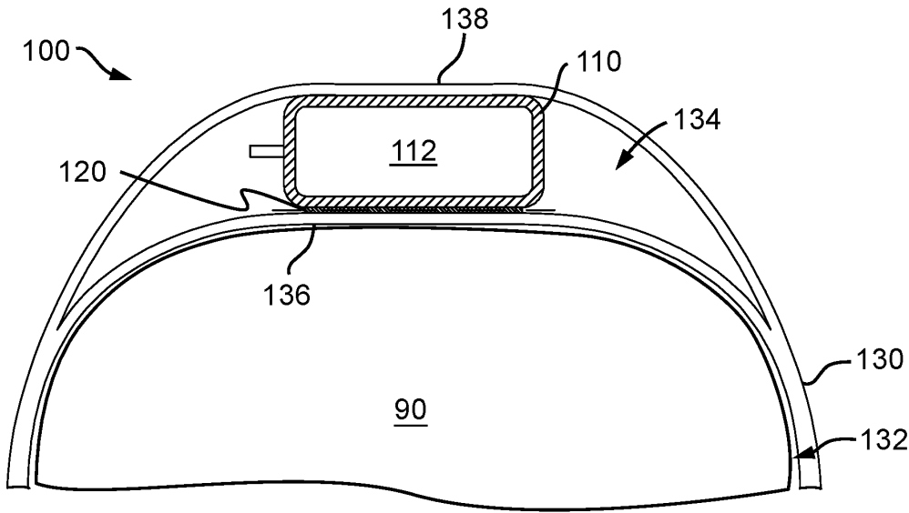
FIG. 3 (VIEW A-A)
