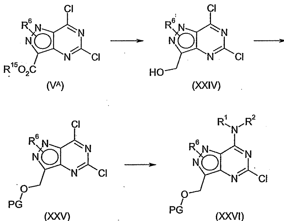
Scheme 25A
