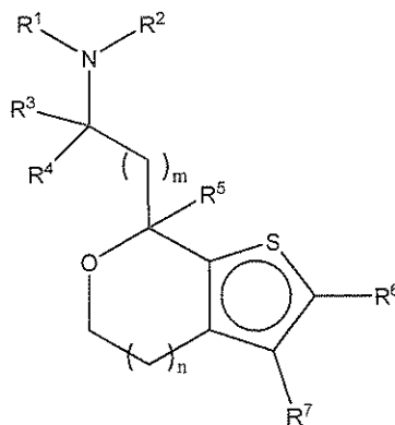
(IVa),
