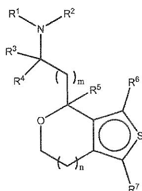
(IIIa),
