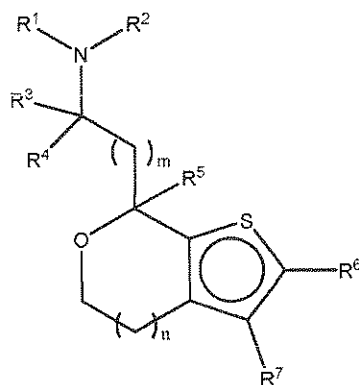
(IVa),
