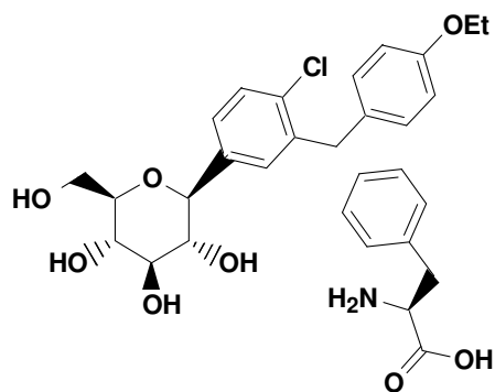
Compound Ik
