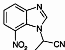
A. 2-(7-nitro-1H-benzimidazol-1-yl)propanenitrile
