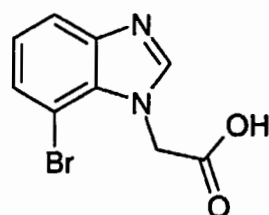
3)(7-Bromo-1H-benzimidazol-1-yl)acetic acid
