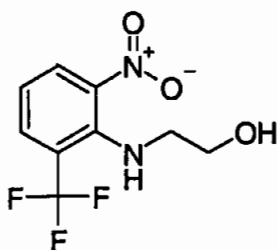
A. 2-[[2-Nitro-6-(trifluoromethyl)phenyl]amino]ethanol
