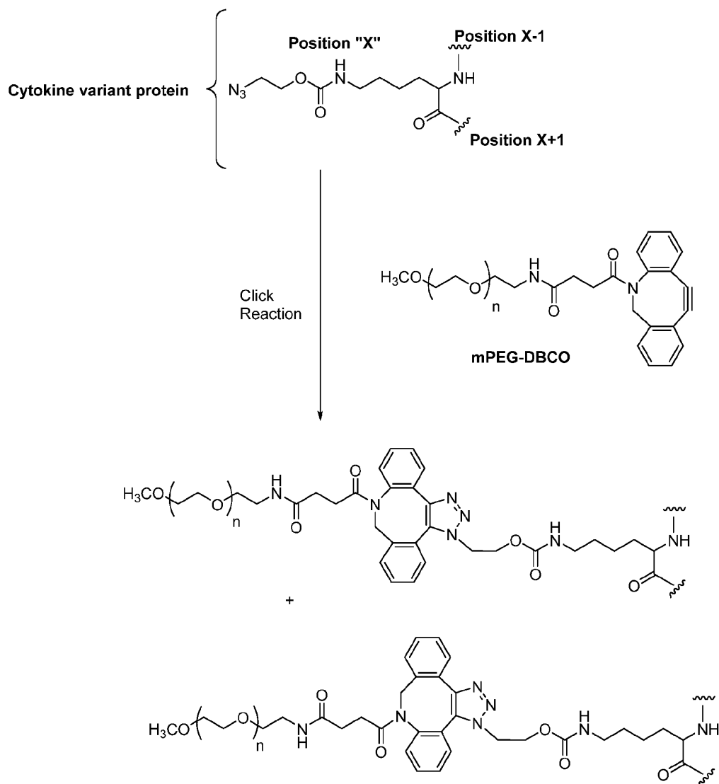
Scheme VI.
