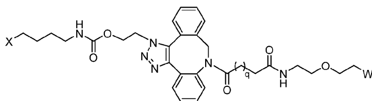
Formula (IVA);
