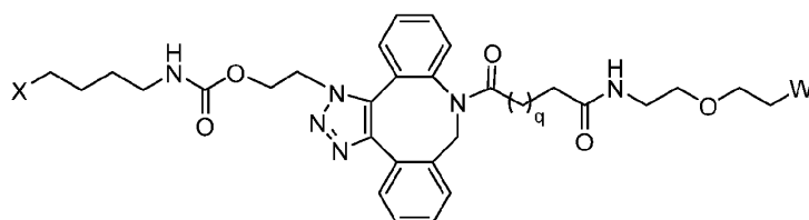
Formula (VA);
