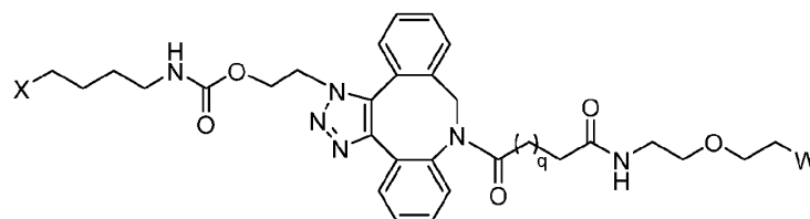
Formula (IVA);
