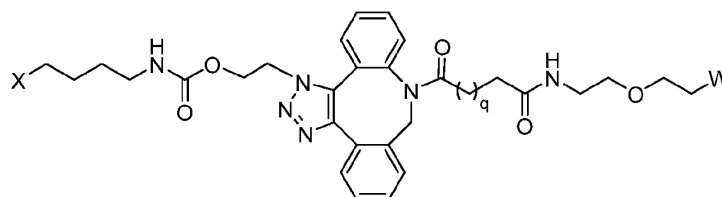
Formula (VA);
