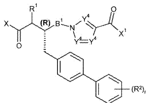
Formula VA
