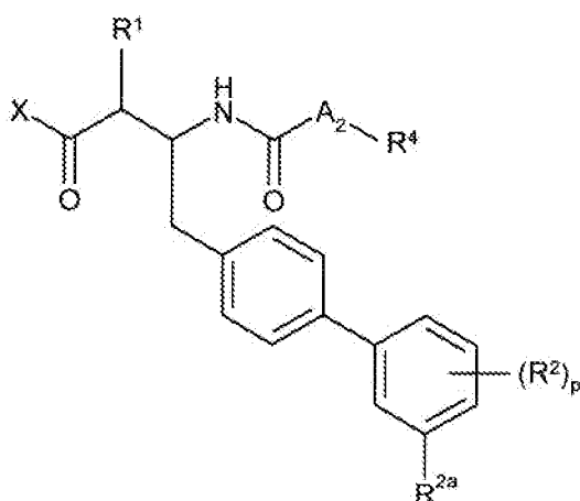
Formula VIIB
