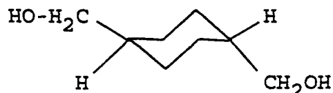
trans -CHDM
