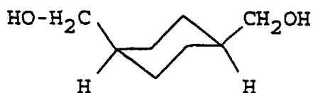
cis -CHDM
