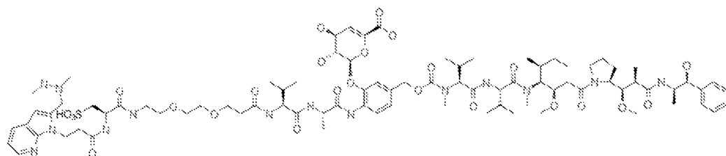
Vlb-82, -18 Da, C 84 H 128 N 14 O 25 S
