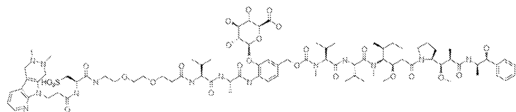
Vlb-82, +12 Da, C 85 H 130 N 14 O 26 S
