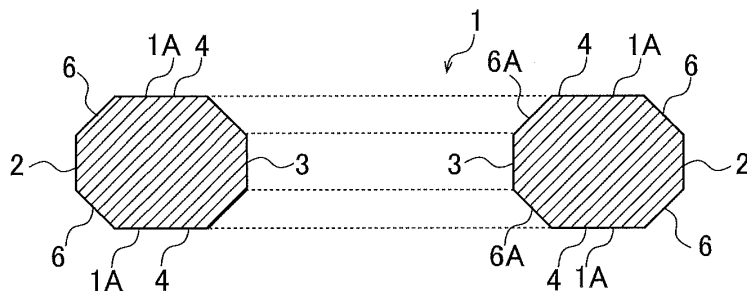
A-A 断面図
