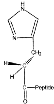
Des-amino-histidyl (DA)-GLP-2
