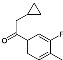
Compound 1-A
