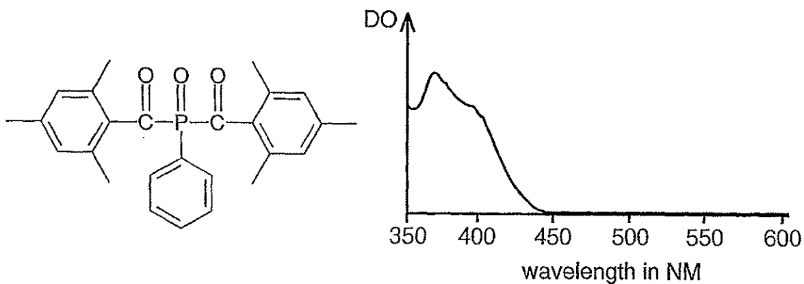
Irgacure 819
