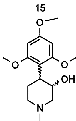
VIII
