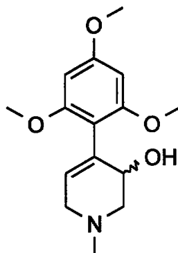
VII
