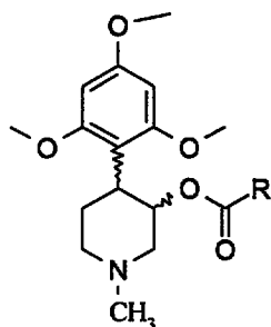
Xa
