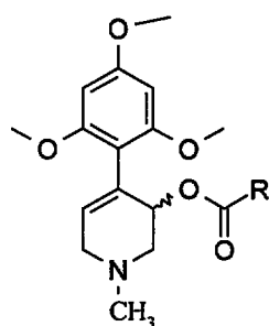
IXa
