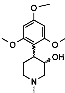
VIII
