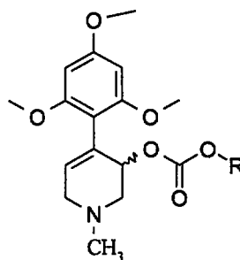
IXb
