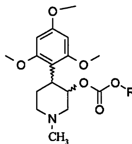
Xb
