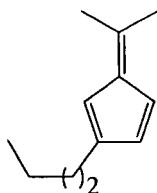
2-(butyl)-6,6-dimethylpentafulvene
