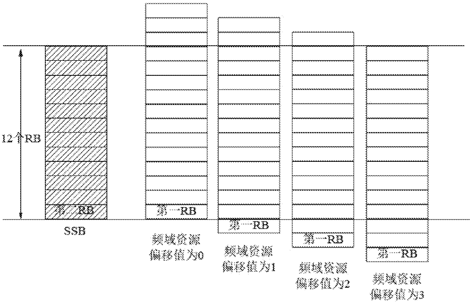
15个RB的CORESET在可用RB数为15的信道中的可能的频域位置
