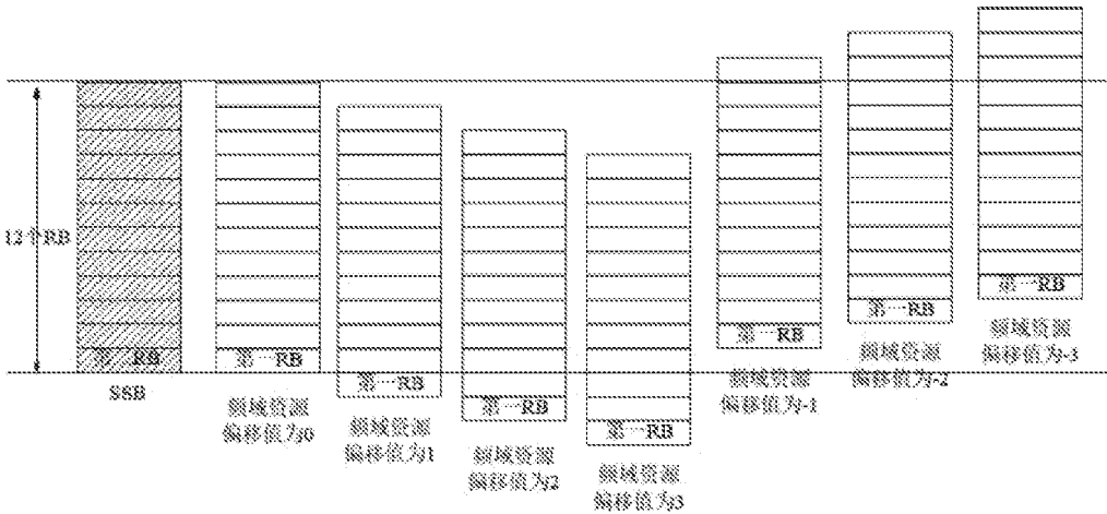
12个RB的CORESET在可用RB数为15的信道中的可能的频域位置
