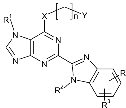
(Vb)
