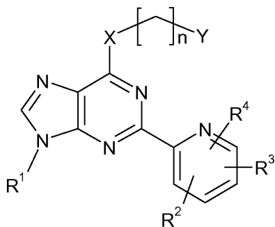
(VIa)
