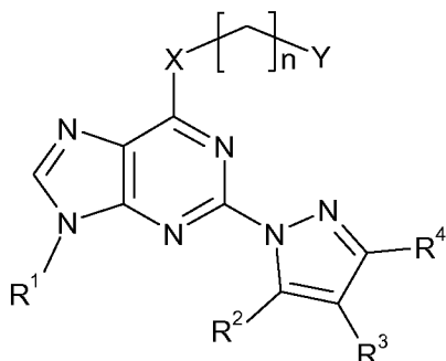
(IIa)
