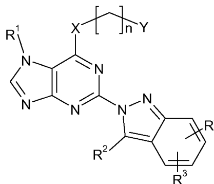
(IIIb)
