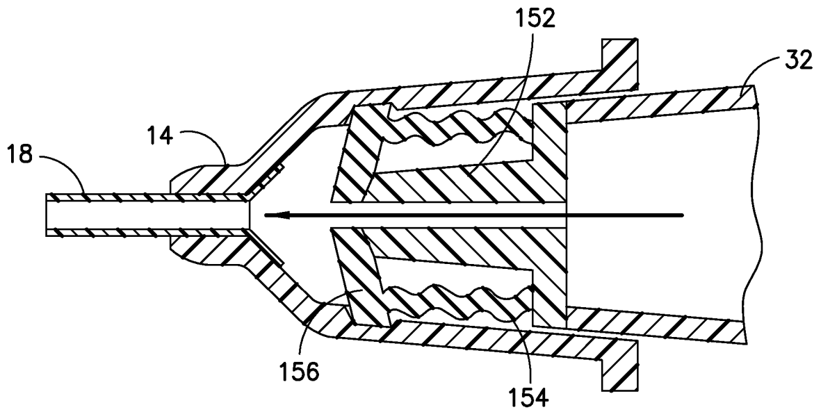
FIG.21A
