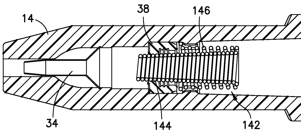
FIG. 19B
