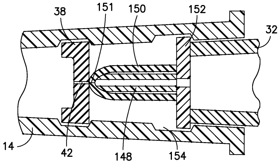
FIG. 20A
