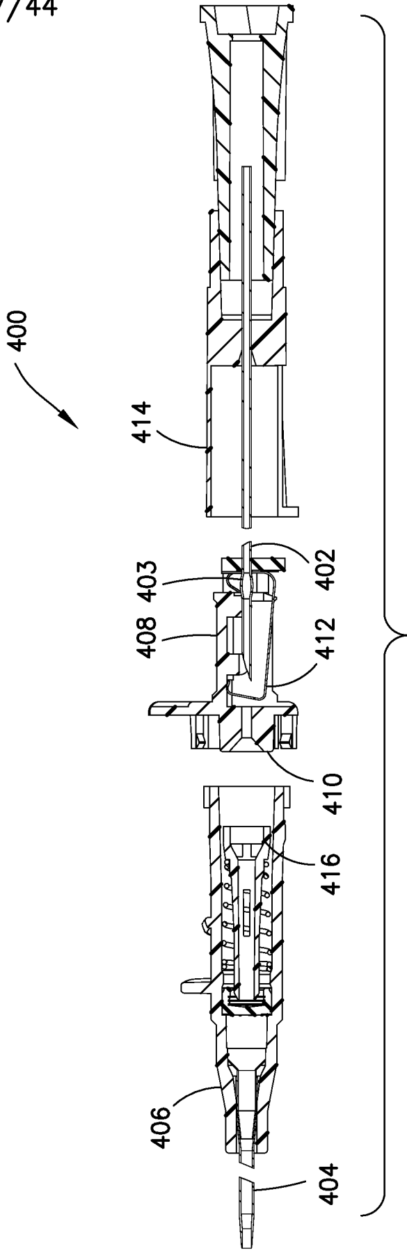
FIG. 44
