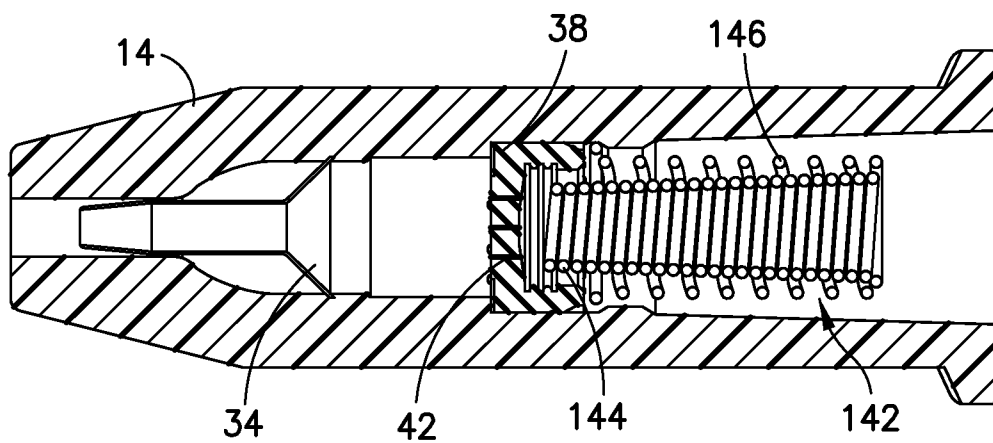
FIG. 19A
