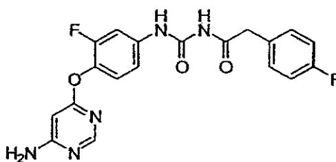
1-(4-(6-Aminopyrimidin-4-yloxy)-3-fluorophenyl)-3-(2-(4-fluorophenyl)acetyl)urea
