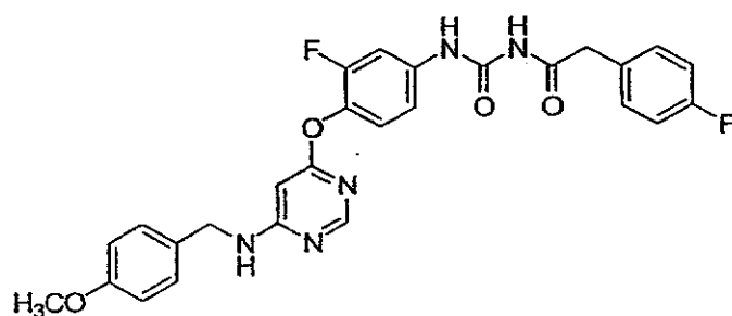
1-(4-(6-(4-Methoxybenzylamino)pyrimidin-4-yloxy)-3-fluorophenyl)-3-(2-(4-fluorophenyl)acetyl)urea
