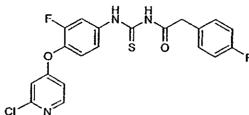
1-(4-(2-Chloropyridin-4-yloxy)-3-fluorophenyl)-3-(2-(4-fluorophenyl)acetyl)thiourea
