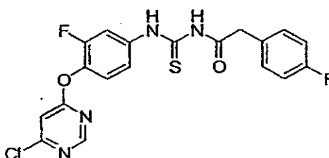
1-(4-(6-Chloropyrimidin-4-yloxy)-3-fluorophenyl)-3-(2-(4-fluorophenyl)acetyl)thiourea
