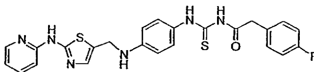
1-(2-(4-Fluorophenyl)acetyl)-3-(4-((2-(pyridin-2-ylamino)thiazol-5-yl)methylamino)phenyl)thiourea
