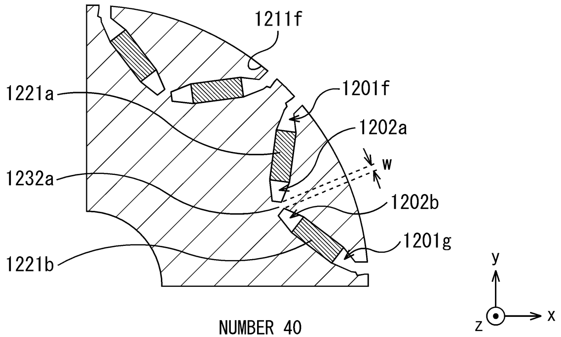
FIG. 12G
