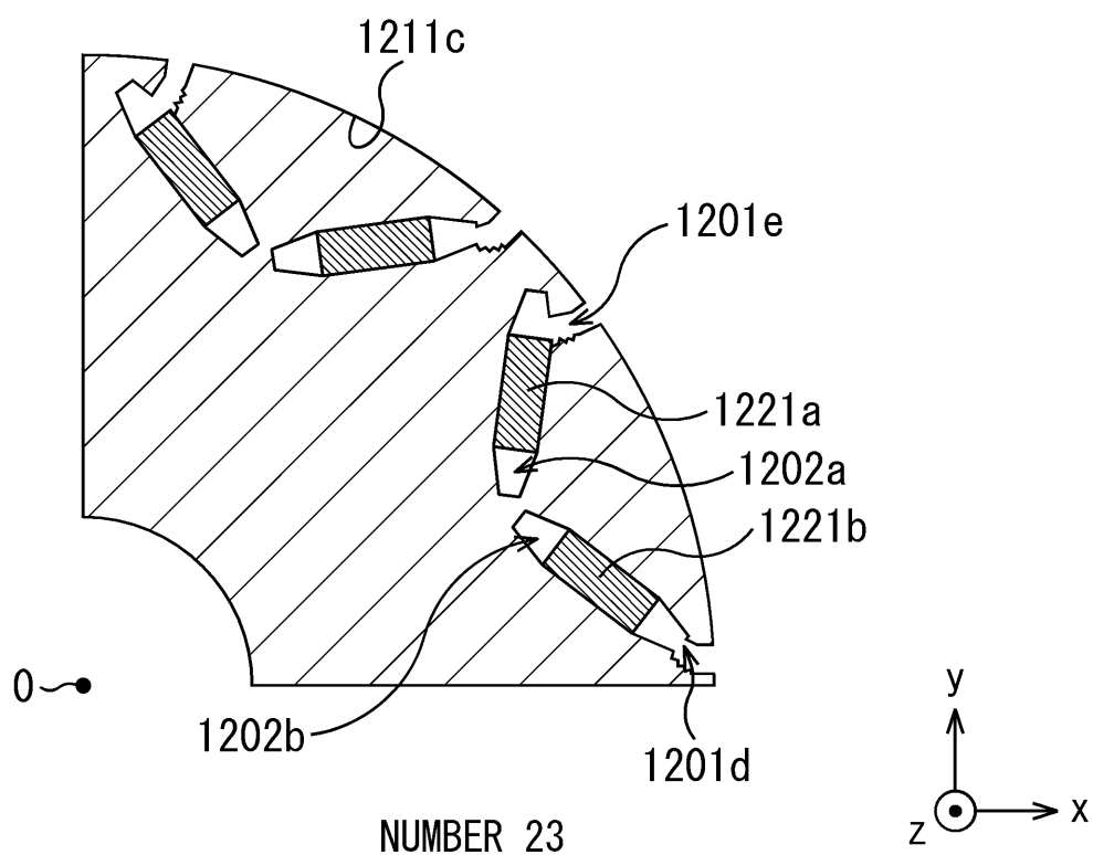
FIG. 12C
