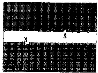
K-selectride
