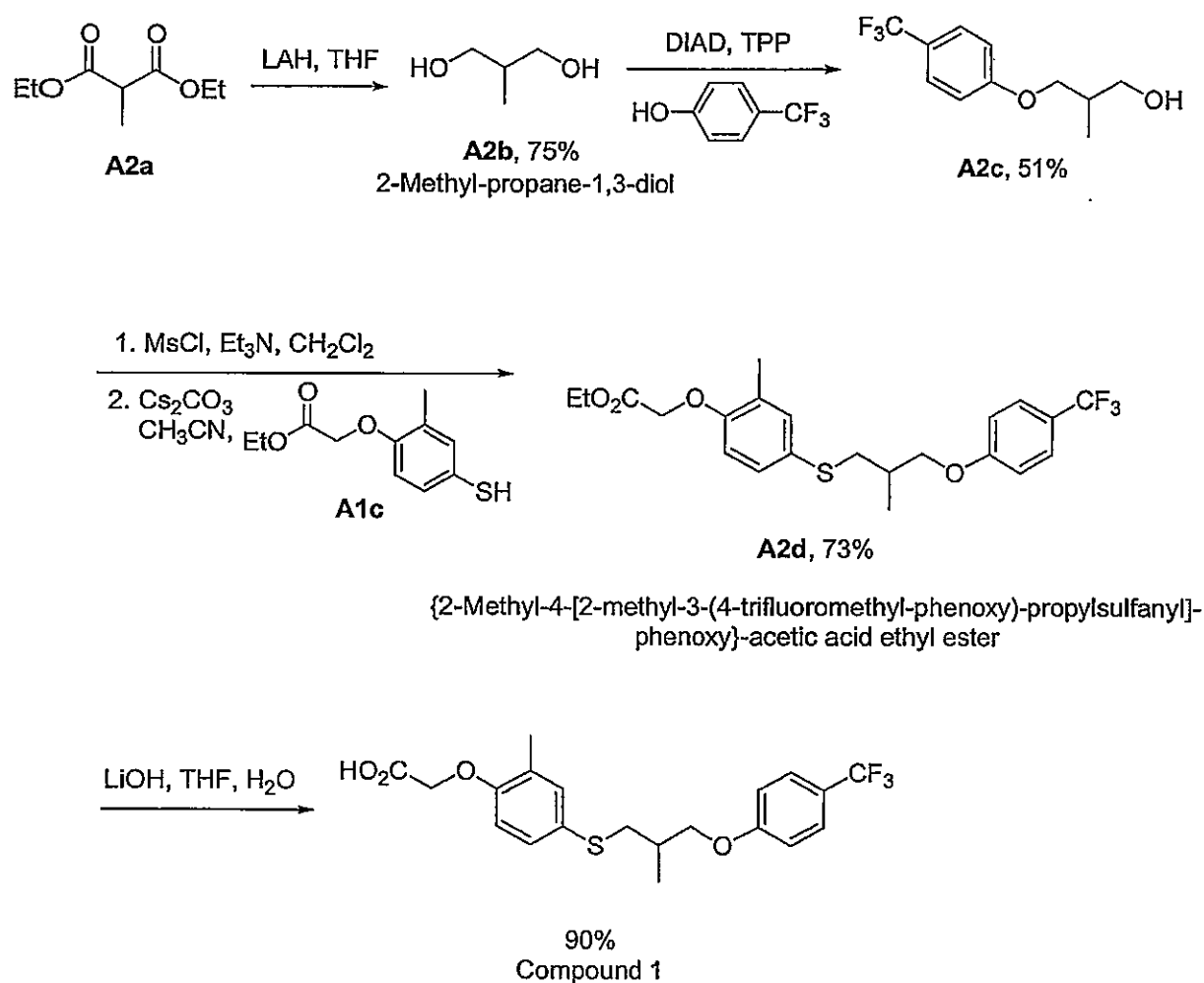
Scheme A2
