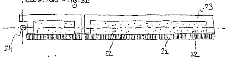
SECTION A-A Fig. 3C
