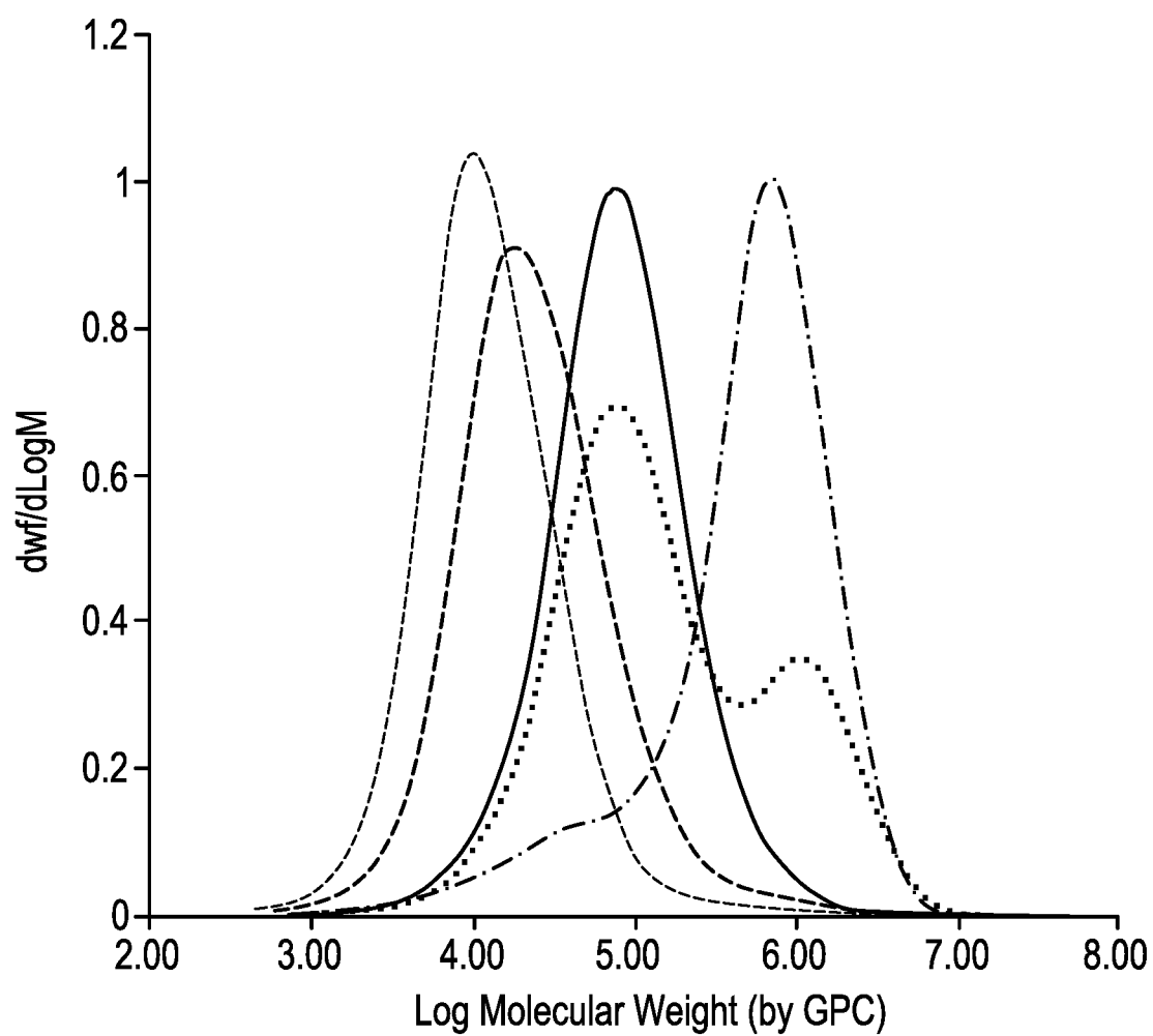
FIG. 3 GPC MWD Overlay
