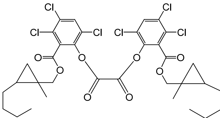
bis(3,4,6-trichloro-2-[[2-butyl-1-methylcyclopropyl)methoxy]carbonyl)phenyl) oxalate
