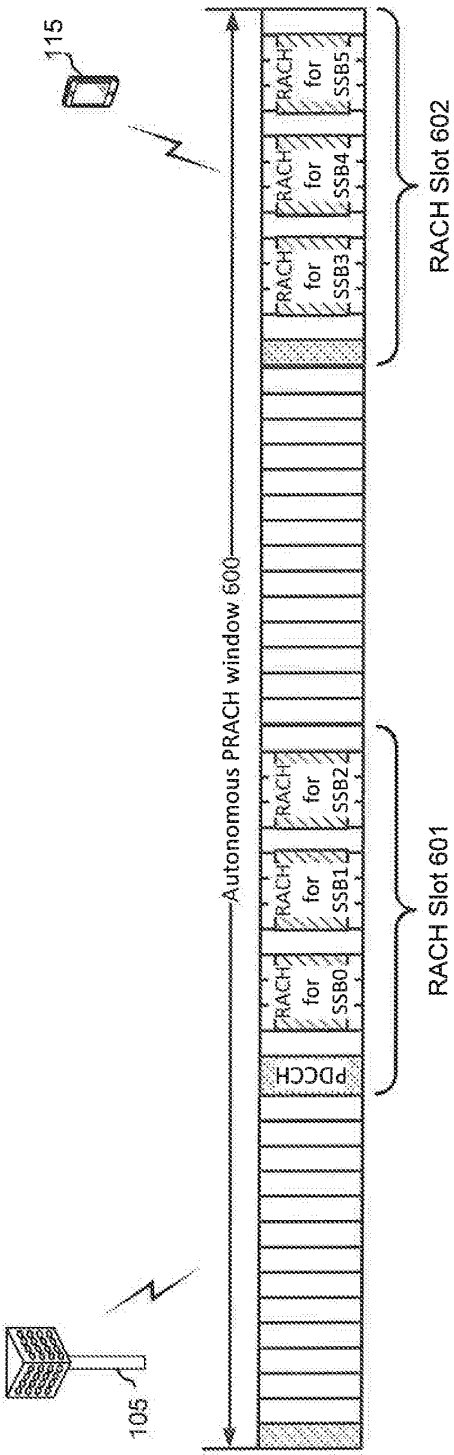
FIG. 6A
