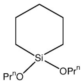
1,1-di-n-propoxy-1-silacyclohexane
