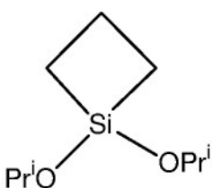
1,1-di-iso-propoxy-1-silacyclobutane
