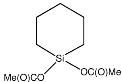
1,1-diacetoxy-1-silacyclohexane
