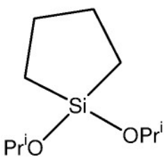
1,1-di-iso-propoxy-1-silacyclopentane
