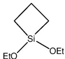
1,1-diethoxy-1-silacyclobutane
