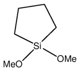
1,1-dimethoxy-1-silacyclopentane
