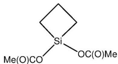
1,1-diacetoxy-1-silacyclobutane
