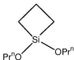
1,1-di-n-propoxy-1-silacyclobutane
