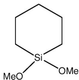
1,1-dimethoxy-1-silacyclohexane
