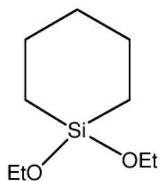
1,1-diethoxy-1-silacyclohexane
