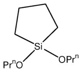
1,1-di-n-propoxy-1-silacyclopentane
