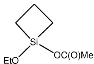
1-ethoxy-1-acetoxy-1-silacyclobutane
