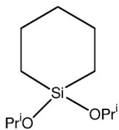
1,1-di-iso-propoxy-1-silacyclohexane
