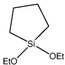
1,1-diethoxy-1-silacyclopentane
