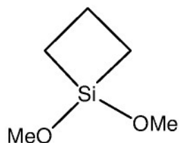
1,1-dimethoxy-1-silacyclobutane
