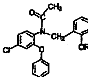
DAA1097 (3) : \text{R}=\text{CH}(\text{CH}_3)_2 [^{11}\text{C}] 3 : \text{R}=\text{}^{11}\text{CH}(\text{CH}_3)_2 [^{11}\text{C}] 7 : \text{R}=\text{}^{11}\text{CH}_2\text{CH}_3 [^{11}\text{C}] 8 : \text{R}=\text{}^{11}\text{CH}_3
